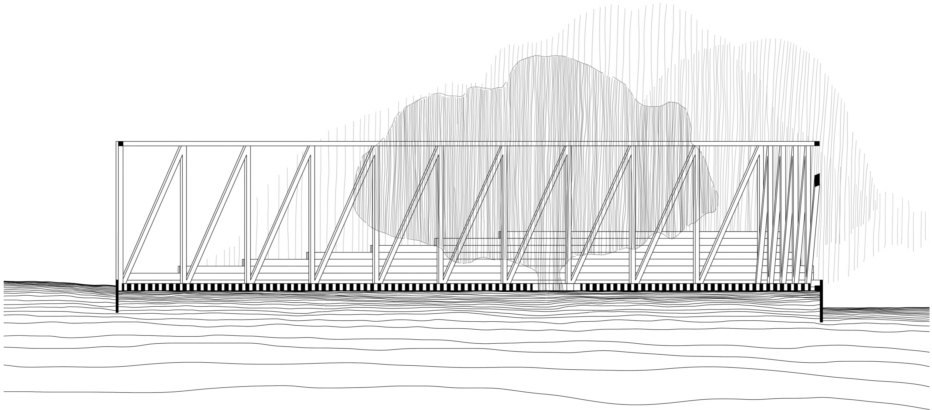
B-B metszet M 1:50
